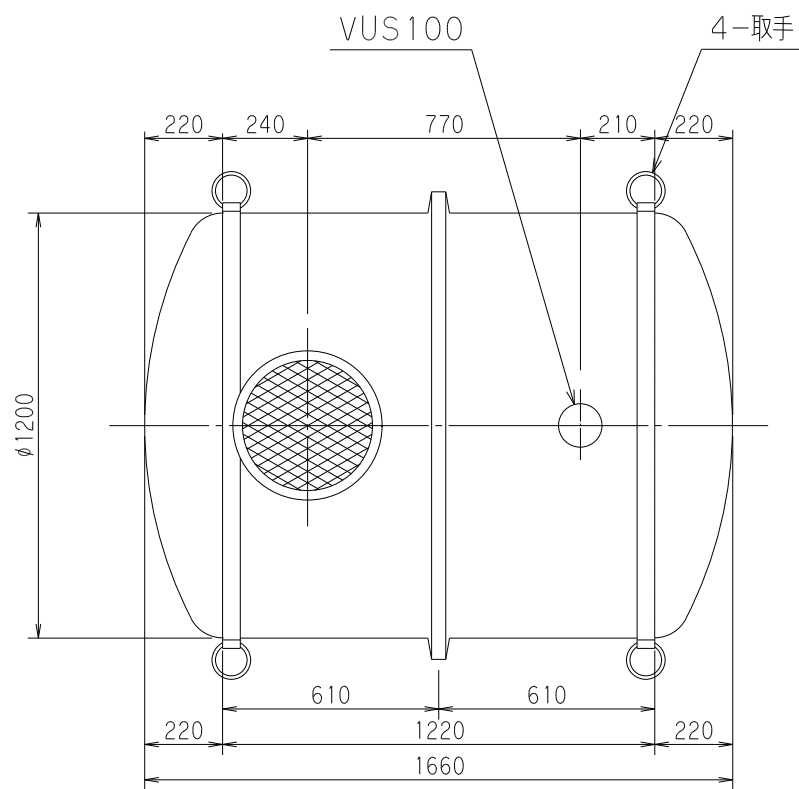
平面図
