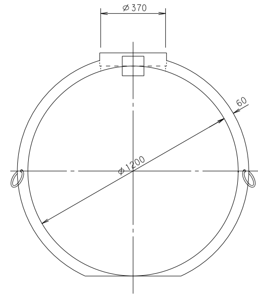
断面図
