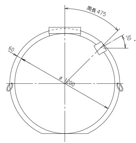
断面図
