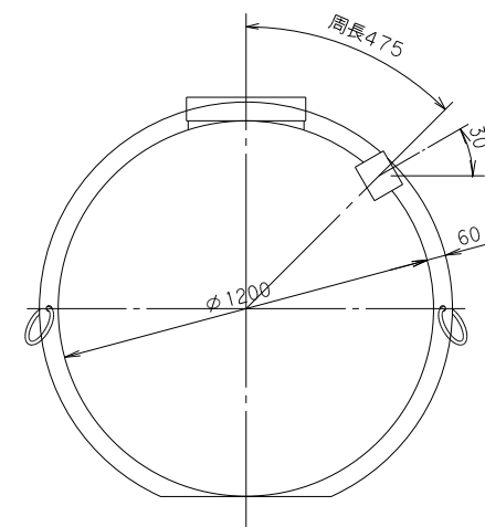
断面図
