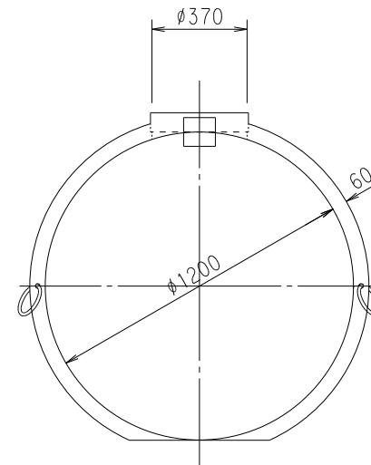
断面図
