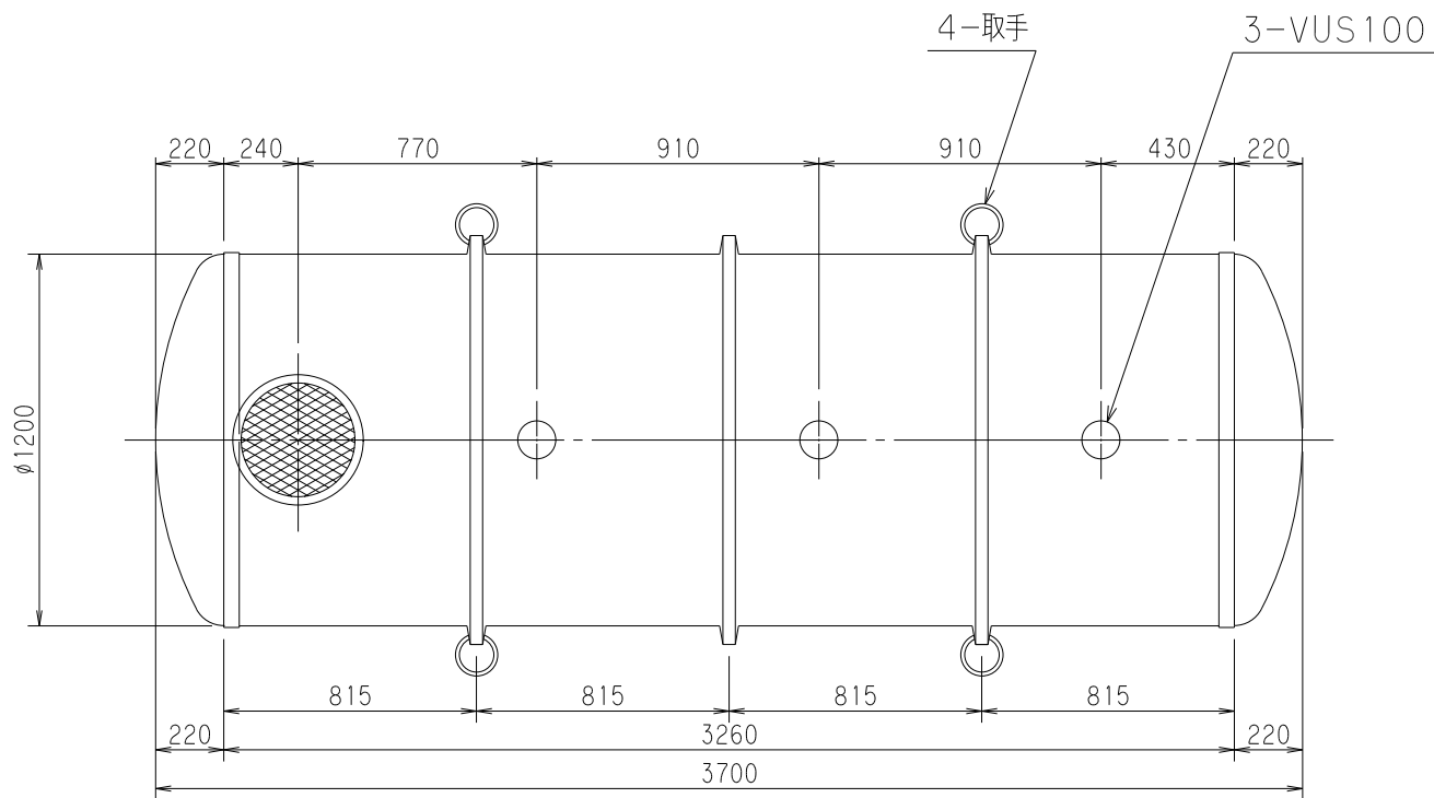
平面図
