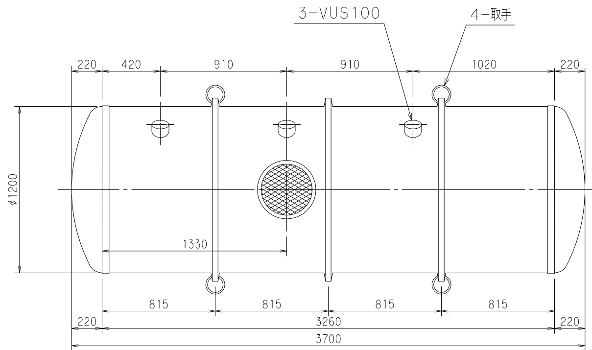
平面図
