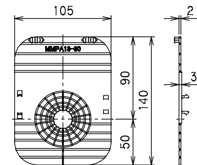
⑤ 土留板
