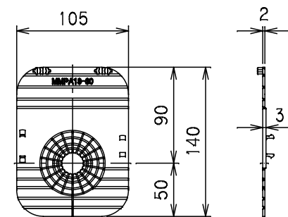
⑤ 土留板
