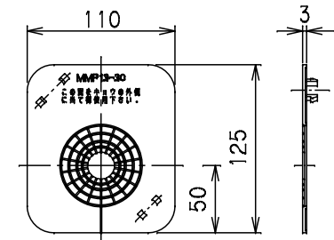
⑦ 土留板
