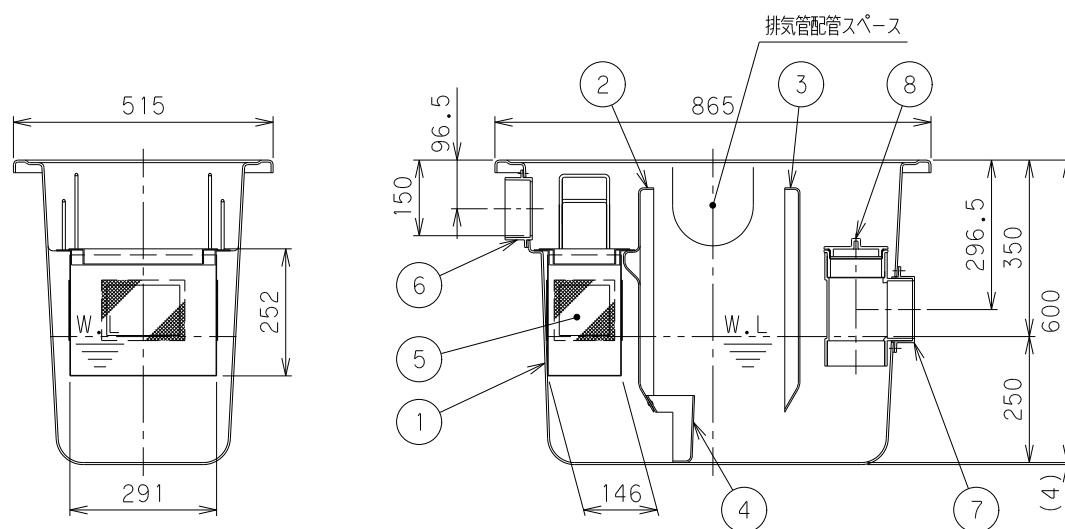
×—×断面图
