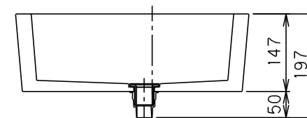
排水栓組立完成図
