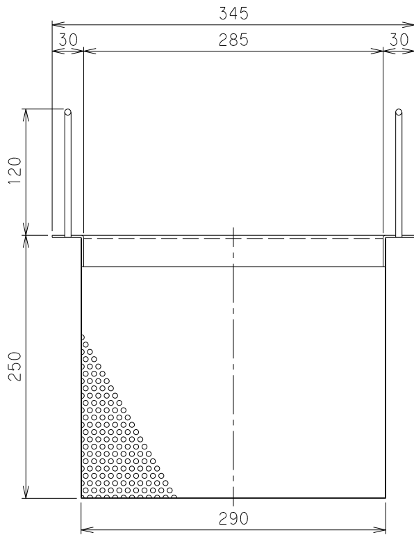
X-X断面
