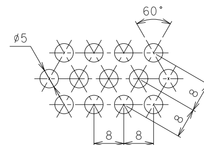
パンチングプレート打抜穴詳細
