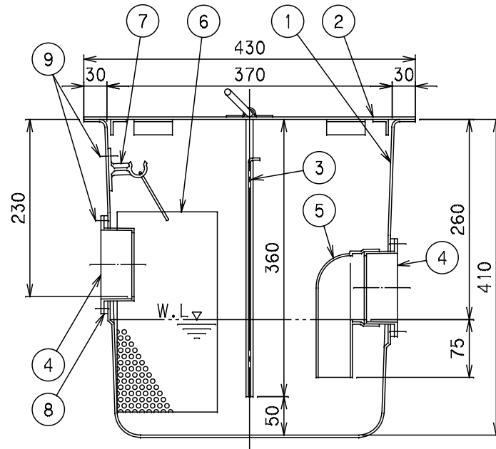
X-X断面図
