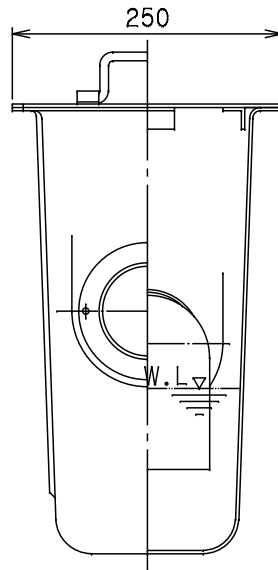
A-A断面図
