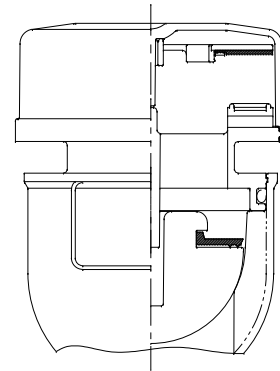
組立図 (開時)
