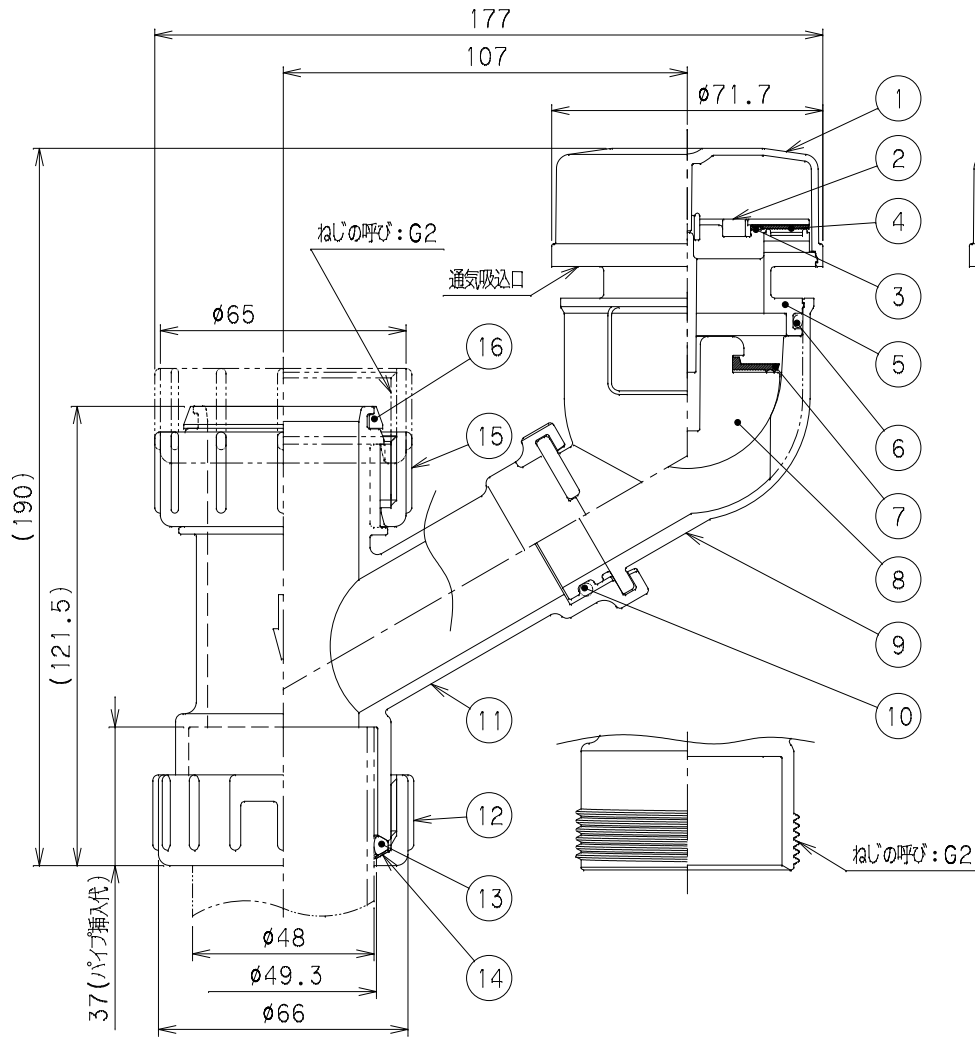
組立図 (閉時)
