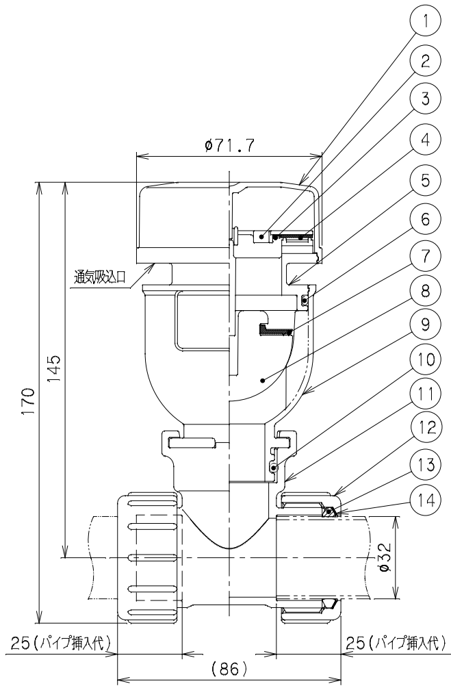
組立図(閉時)
