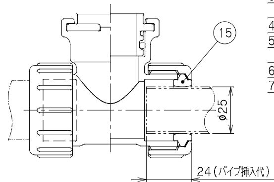
呼び径25
