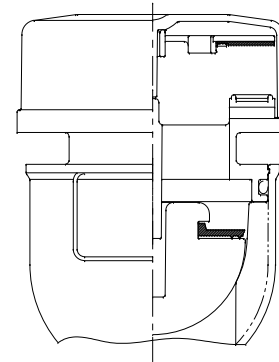
組立図(開時)
