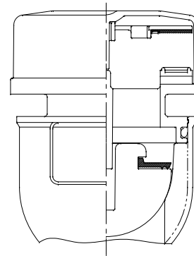
組立図(開時)
