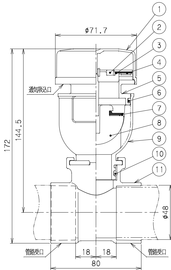
組立図(閉時)
