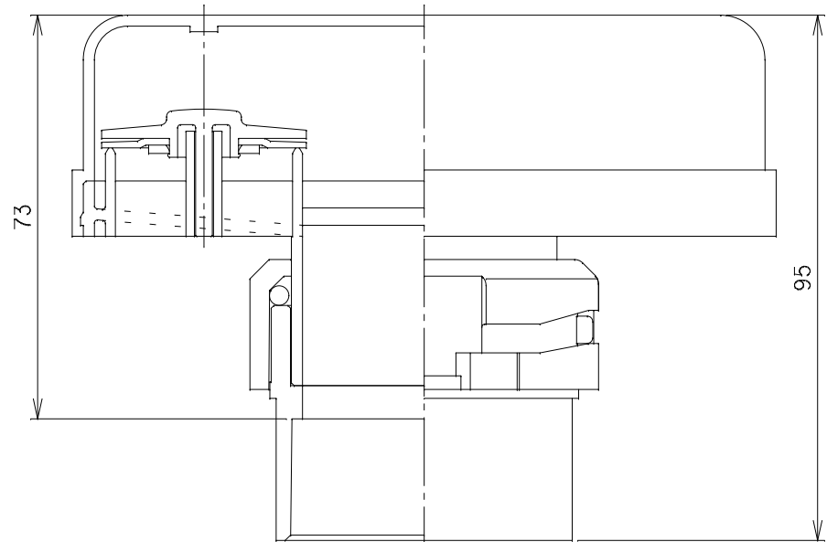
組立図
