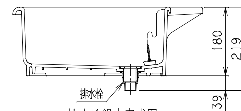
排水栓組立完成図
