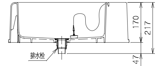
排水栓組立完成図
