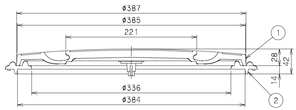
X-X断面図
