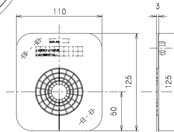
⑥ 土留板
