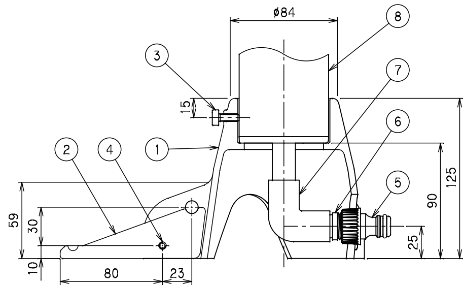
A-A' 断面図
