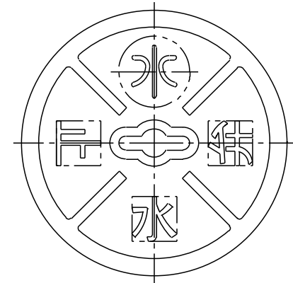
蓋平面図
