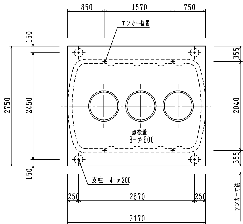
スラブ平面図 S = 1/50
