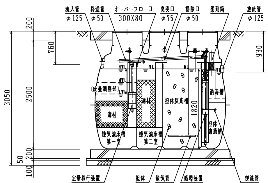
断面図 S = 1/50
