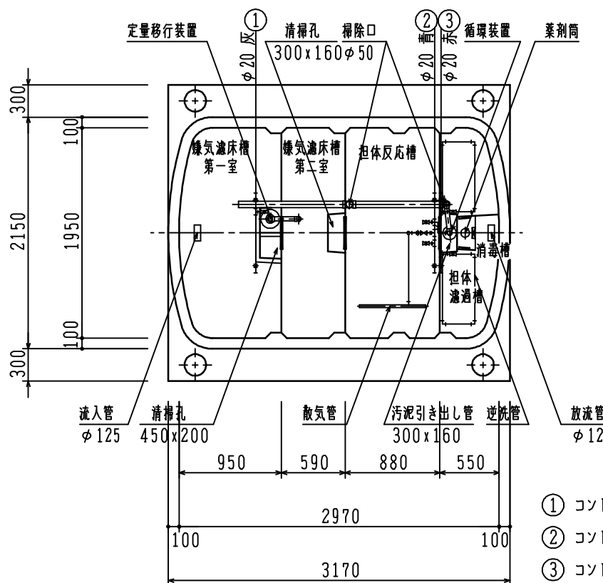
平面図 S = 1/50
