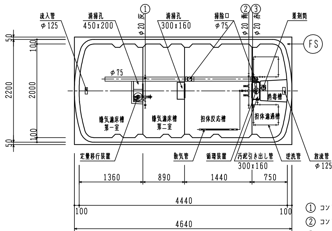
平面図 S = 1/50
