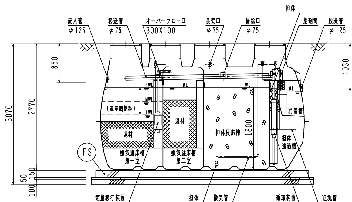
断面図 S = 1/50
