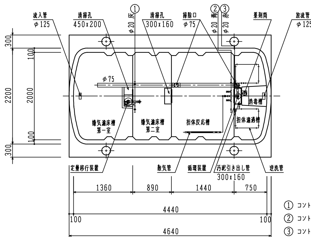
断面図 S = 1/50
