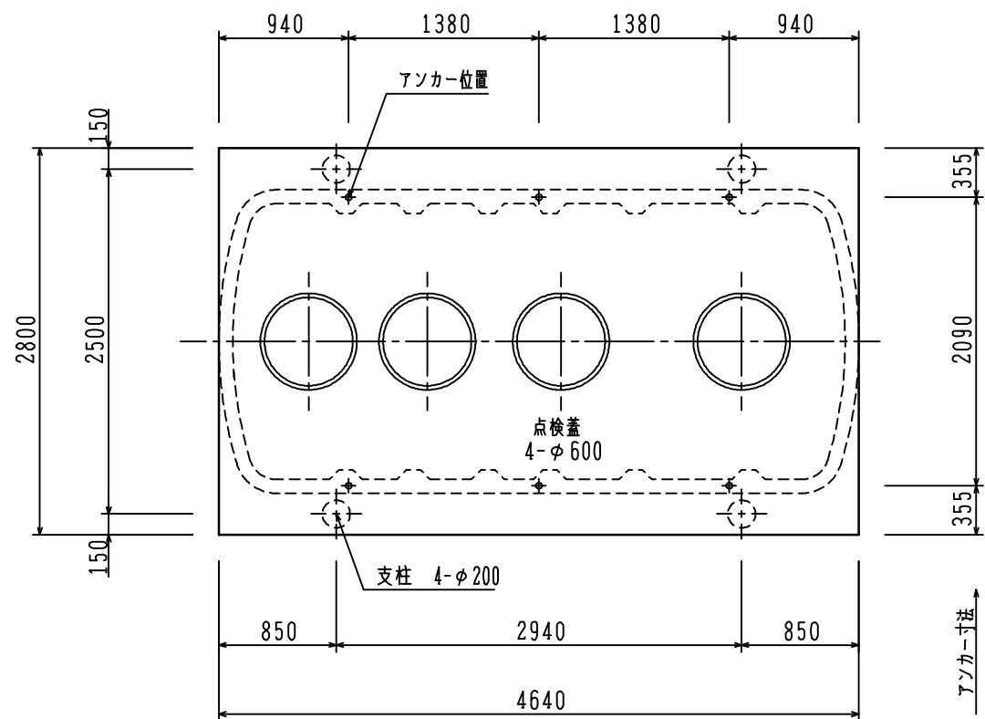
スラブ平面図 S = 1/50
