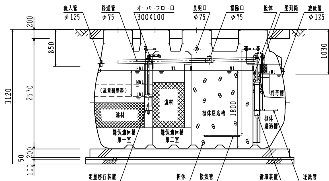
断面図 S = 1/50
