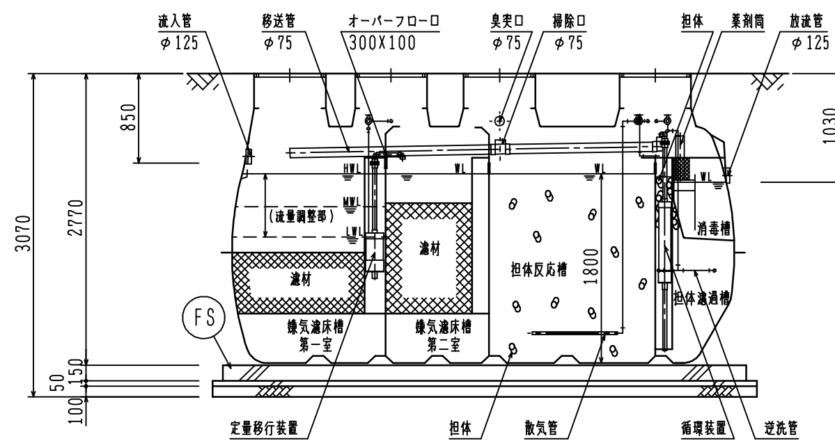
断面图 S = 1/50
