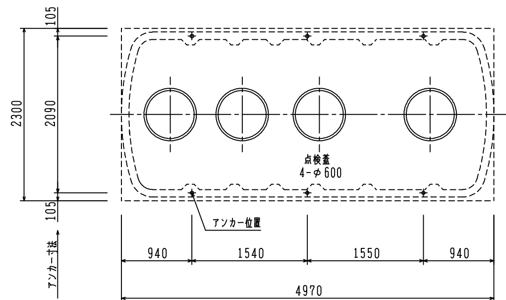
スラブ平面図
