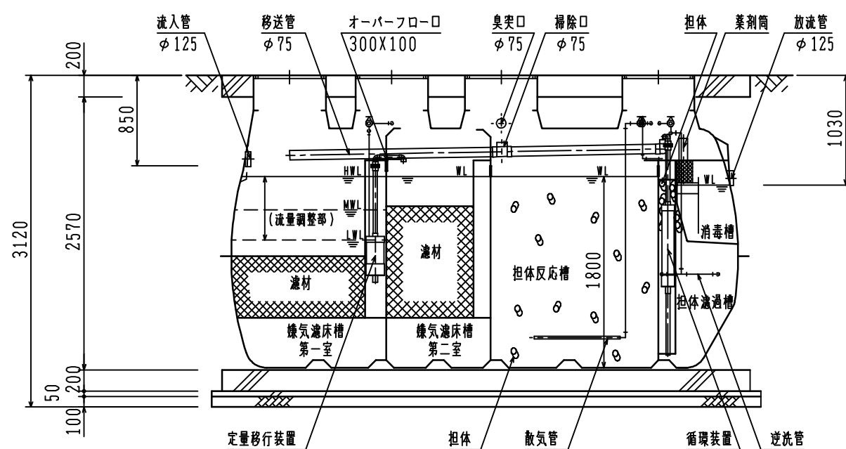
断面図 S = 1/50
