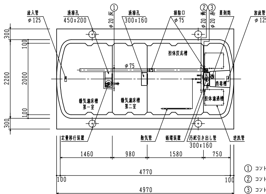
断面図 S = 1/50
