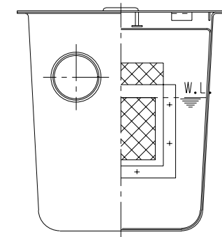
O-Z断面
