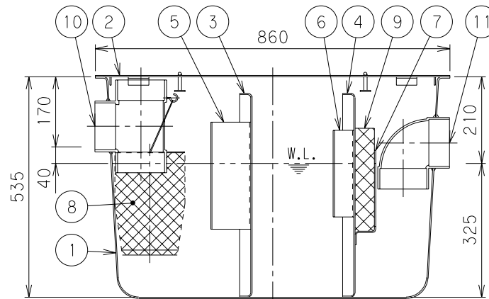
X-X断面
