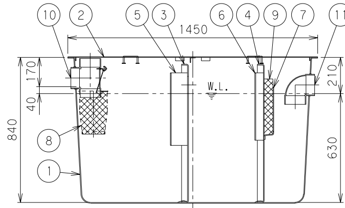
X-X断面
