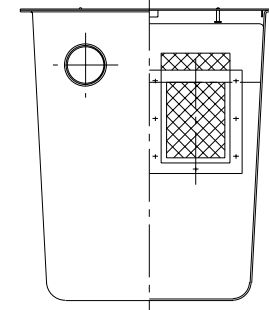
O-Z断面
