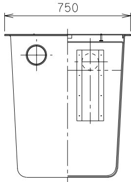
O-Y断面
